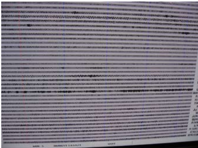
Zapis sejsmografu
